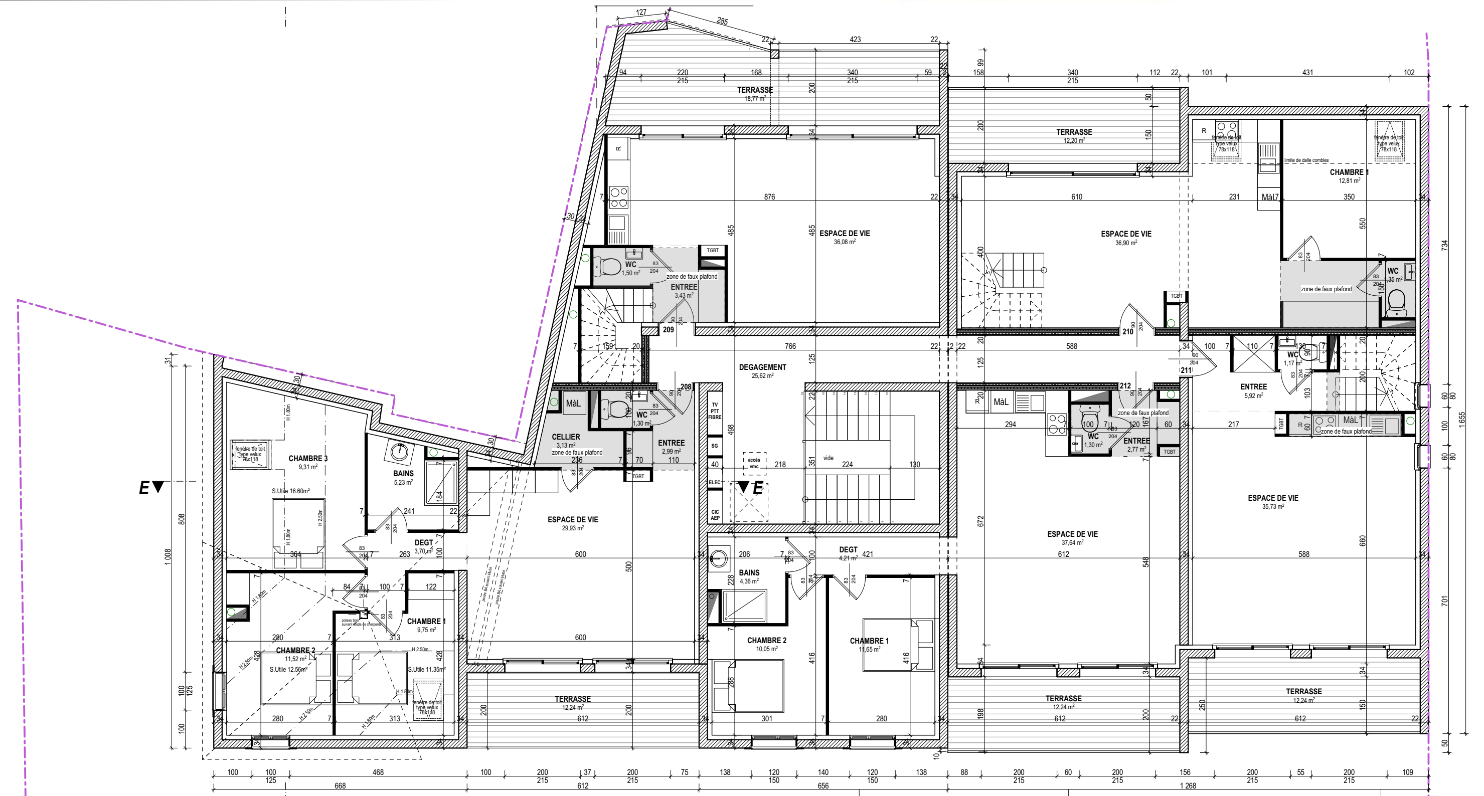
ETAGE 2_1/100
