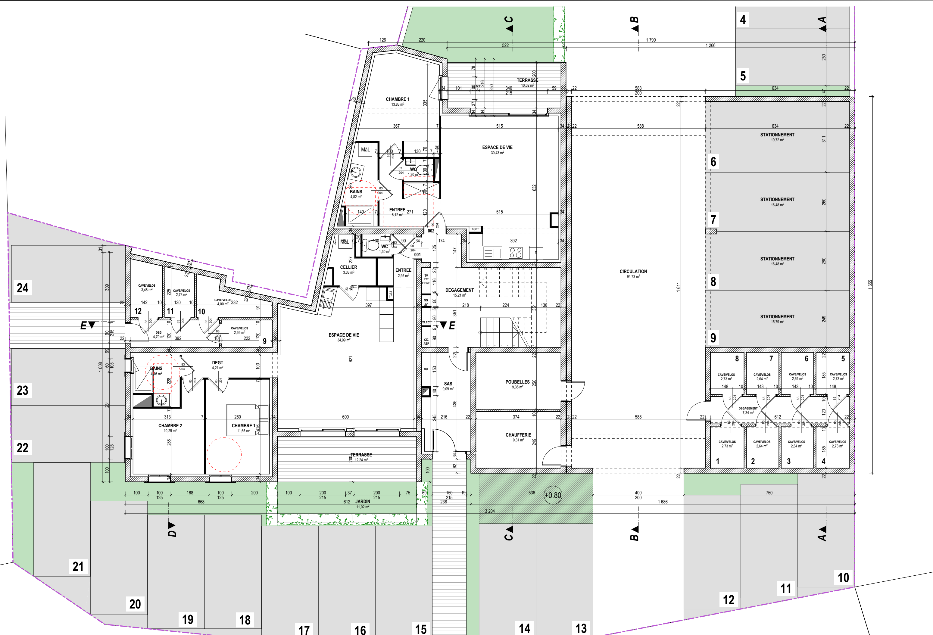
RDC_1/100
