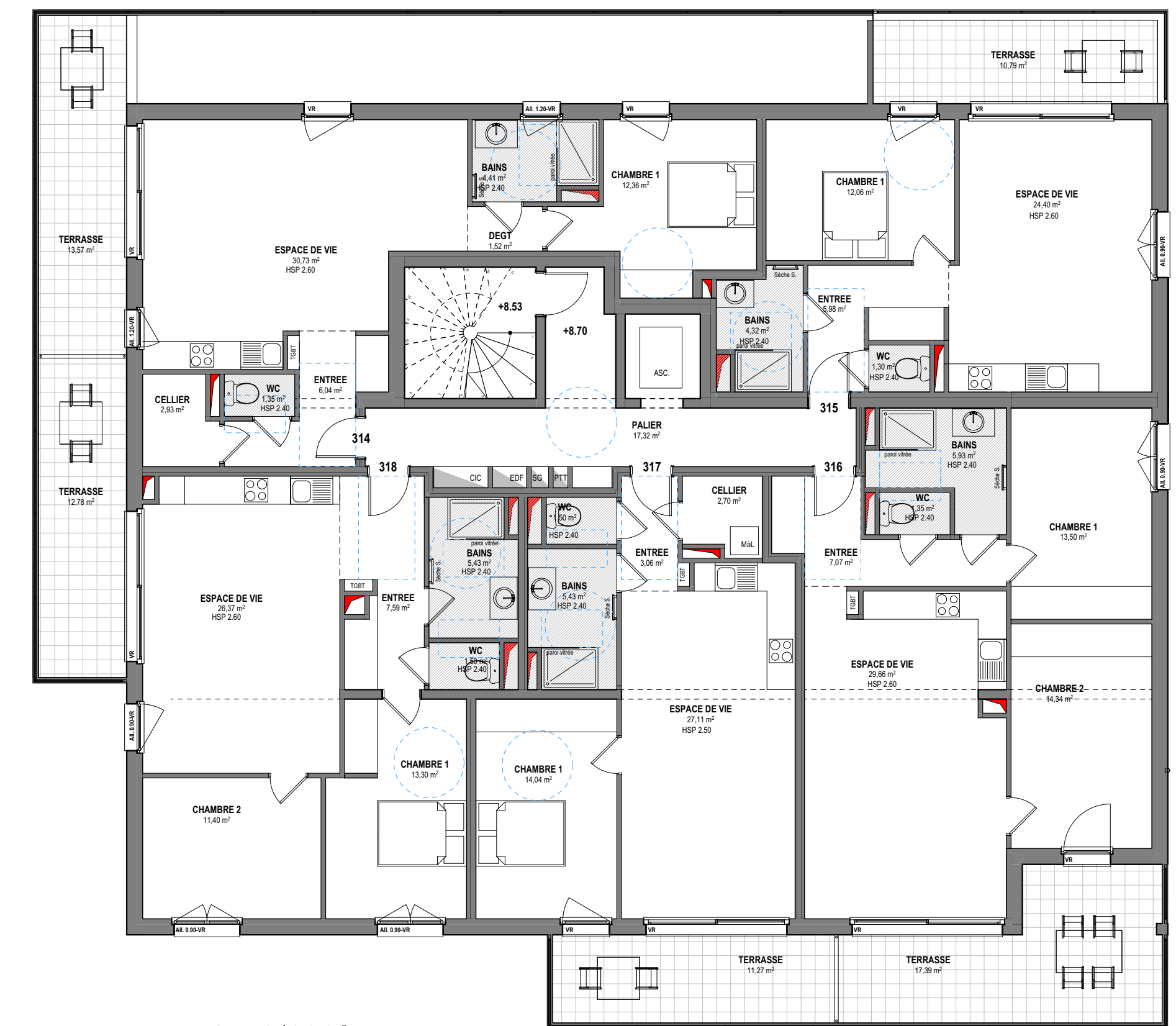
Etage 3 - 1/100ème
