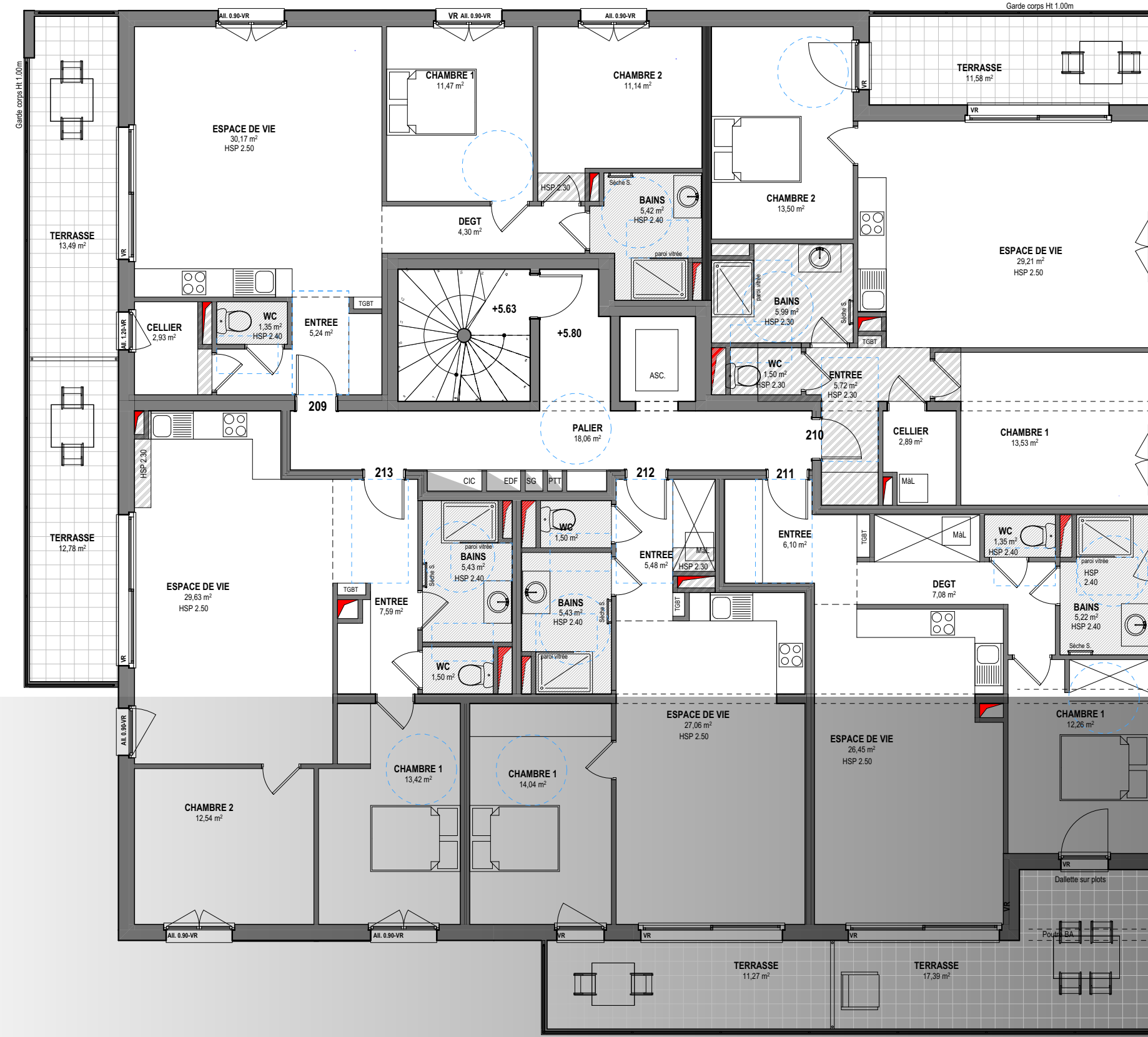
Etage 2 - 1/100ème
